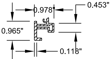
⑪ TRANSOM ALUM. REINF.-612428
